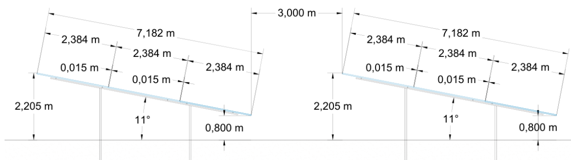
Abbildung 3: Zeichnung der Unterkonstruktion (Quelle: Auftraggeber)
